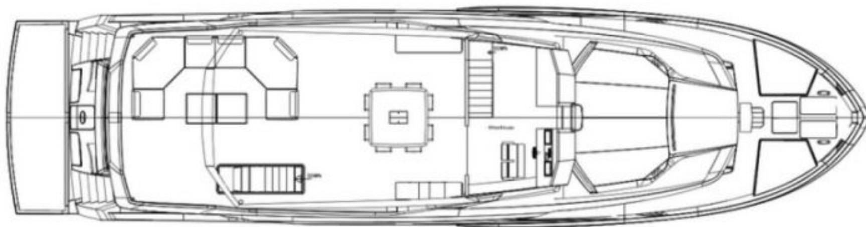
Flybridge
